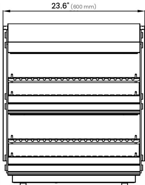
ITEM 47510 • 24" WARMER
